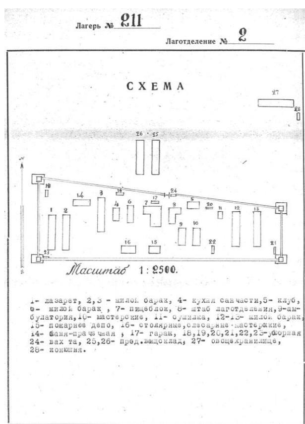
Фото 1. Схема и характеристика 2-го лаготделения лагеря № 211 при Архангельском целлюлозно-бумажном комбинате. 7 февраля 1947 г.
